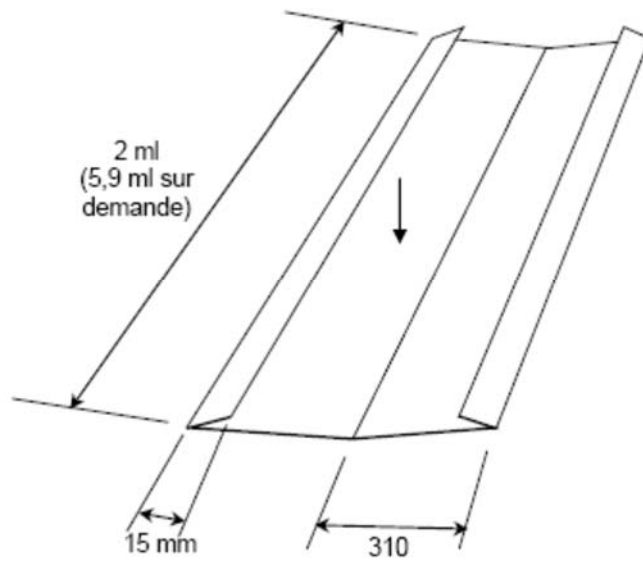
Figure 9 – Bande de noue
