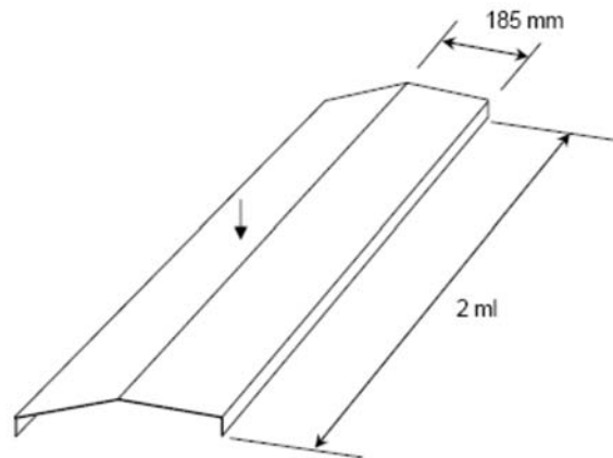
Figure 6 – Bande de faitage simple
