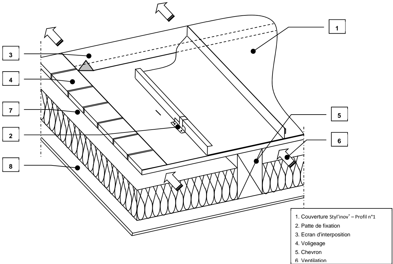
Figure 18 – Écran d'interposition – Styl'inov® – Profil n° 1
