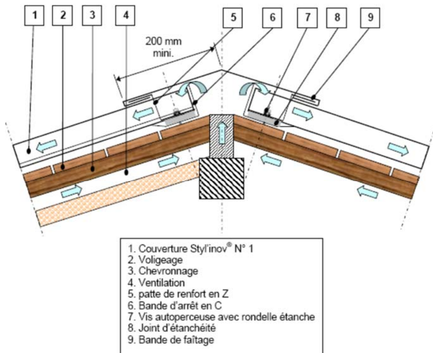
Figure 13b – Faitage ventilé (pente > à 7 %)
