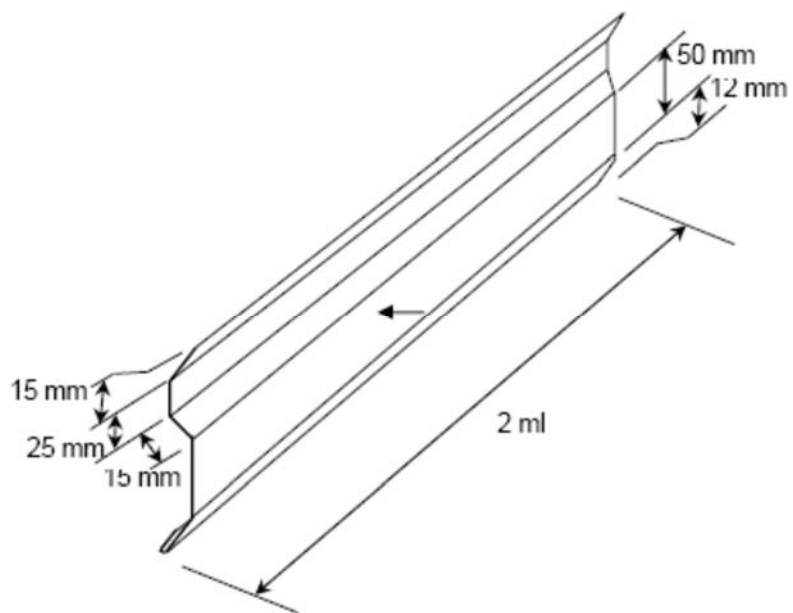
Figure 10 – Bande solin pour joint mastic
