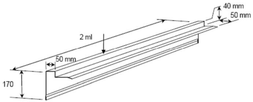
Figure 8 – Bande de rive simple
