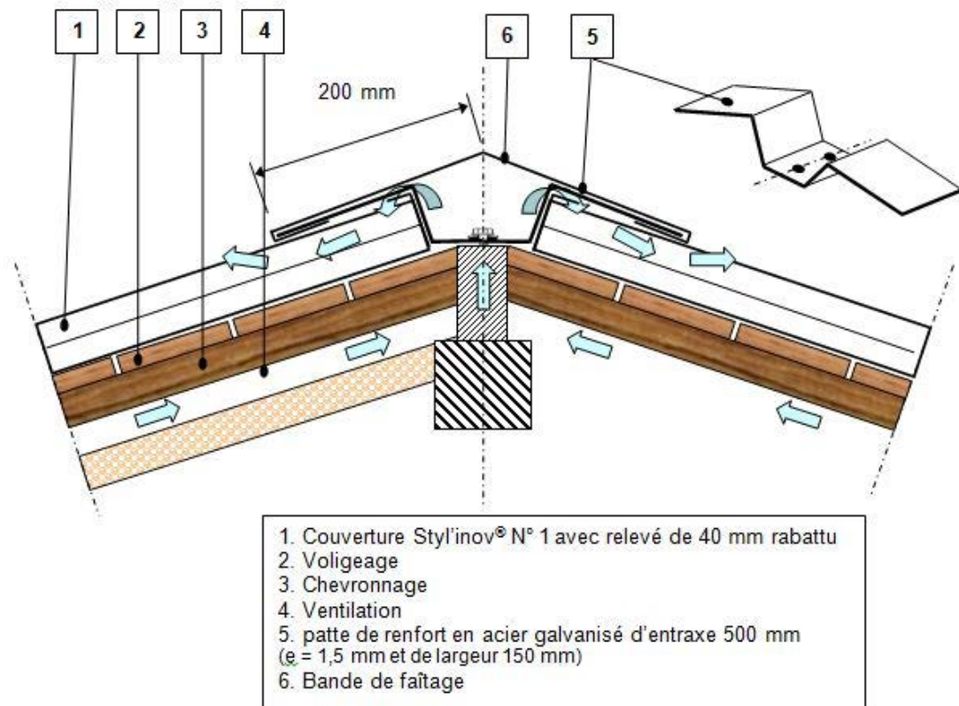
Figure 13a – Faitage ventilé (pente mini 5 %)
