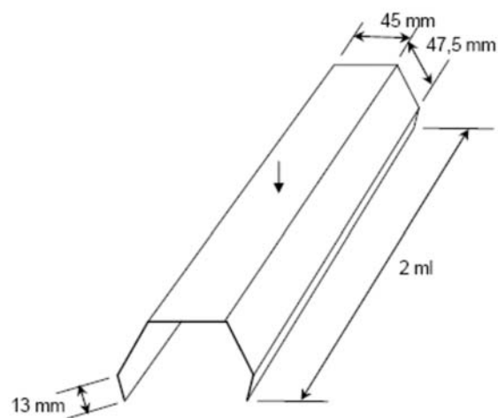
Figure 6 – Bande de faitage simple
